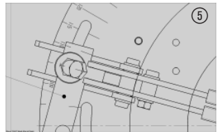
Brake
